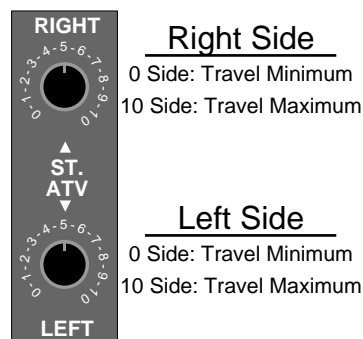
(Steering ATV)
